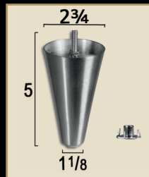
4913* Du Pont Vanity Leg 5 x 2¾
